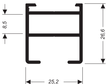
SU-091 0,401 kg/m
