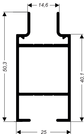
SU-190 0,553 kg/m
