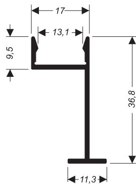
TMR-1447 0,252 kg/m
