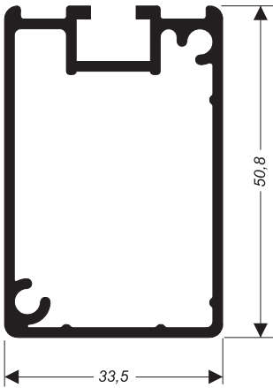
CG-077 0,732 kg/m
