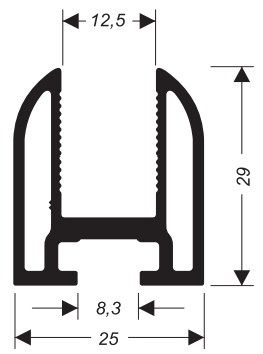
CEG-018 0,625 kg/m
