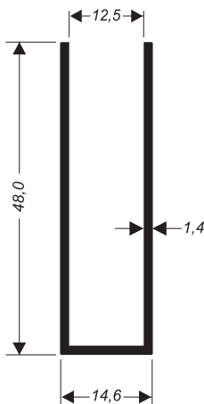
U-580 (AL-335) 0,350 kg/m
