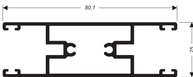
MN-027 0,978 kg/m
