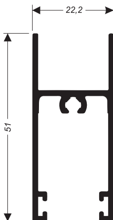
SU-187 0,512 kg/m
