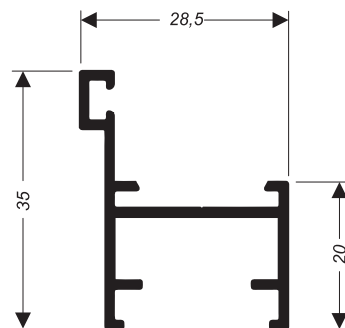
SU-079 (CX-342) 0,297 kg/m
