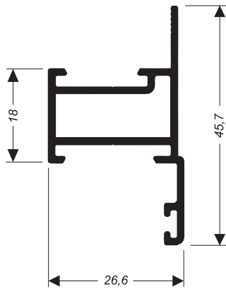
SU-200 (CX-148) 0,404 kg/m
