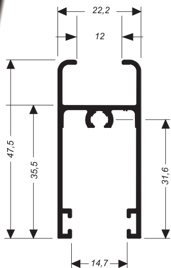
SU-186 0,507 kg/m
