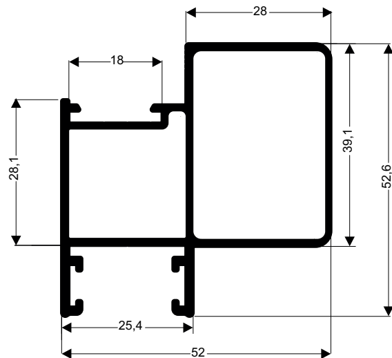
SU-044 0,981 kg/m
