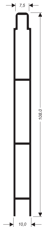
GS-034 0,672 kg/m
