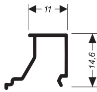
SU-102 (CX-144) 0,100 kg/m
