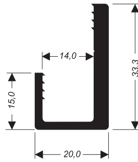
CG-075 0,521 kg/m
