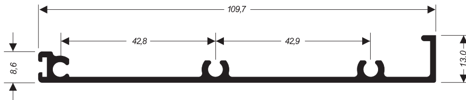
MN-002 0,700 kg/m
