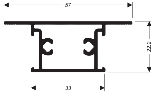
SU-227 (CX-344) 0,544 kg/m
