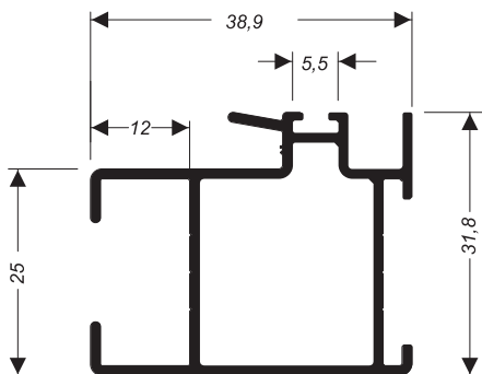
SU-056 0,539 kg/m
