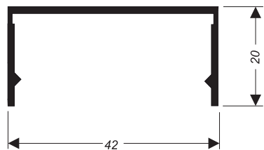
IFC-013 (U-621) 0,265 kg/m
