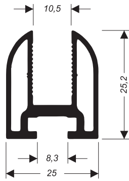
CEG-016 0,595 kg/m
