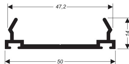
U-878 0,385 kg/m
