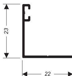
CX-1006 0,138 kg/m
