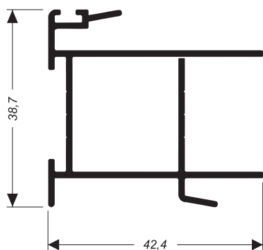
SU-069 (CX-339) 0,536 kg/m
