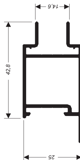
SU-192 (CX-153) 0,475 kg/m
