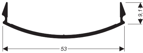
CG-074 0,239 kg/m
