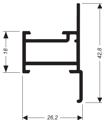
SU-081 (CX-150) 0,364 kg/m
