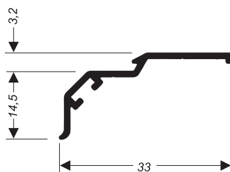
SU-083 (L-794) 0,145 kg/m
