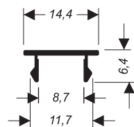
BX-105A 0,065 kg/m
