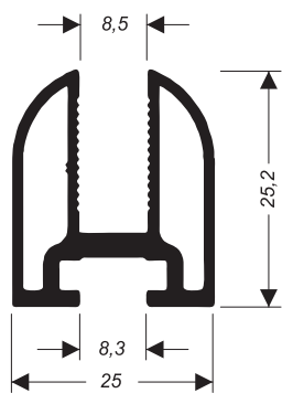
CEG-015 0,594 kg/m
