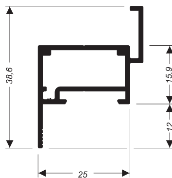
SU-098 0,401 kg/m
