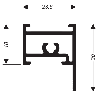
SU-082 (CX-151) 0,345 kg/m
