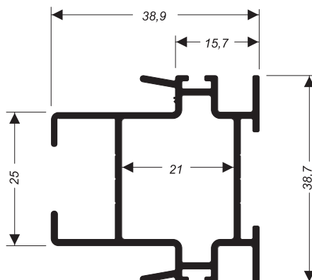
SU-057 0,631 kg/m
