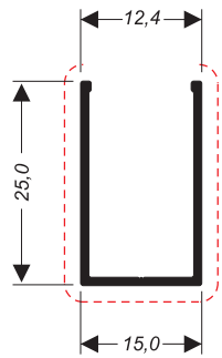
U-555L 0,171 kg/m
