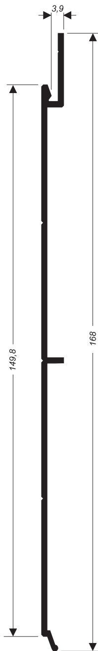
Y-335 0,610 kg/m
