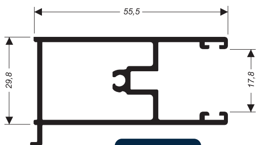
MN-007 0,661 kg/m
