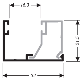
BX-291 (BX-101) 0,220 kg/m
