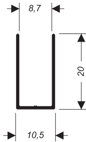
BX-110L 0,119 kg/m
