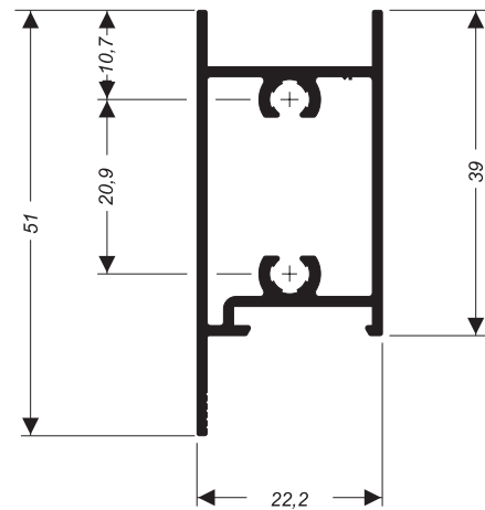
SU-110 0,534 kg/m
