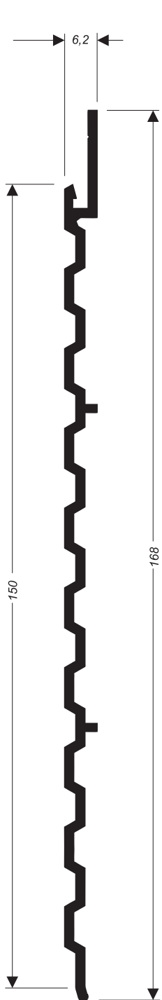
Y-355 0,680 kg/m
