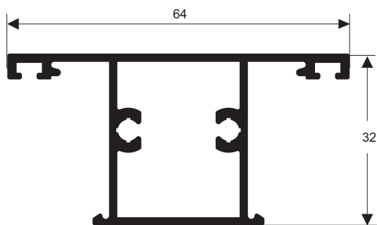
LG-074 0,734 kg/m
