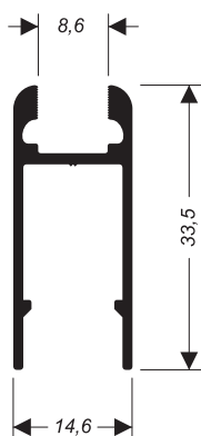
CX-1008 0,307 kg/m
