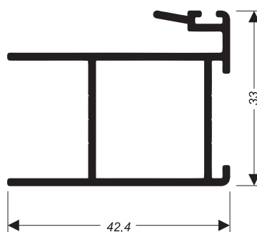
SU-070 (CX-340) 0,486 kg/m
