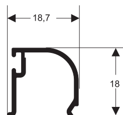
LG-164 0,160 kg/m
