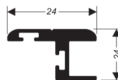
Y-343 0,271 kg/m
