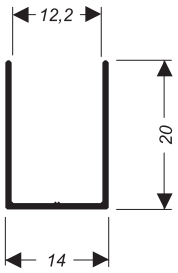
BX-037L 0,127 kg/m
