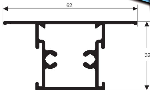
LG-079 0,753 kg/m
