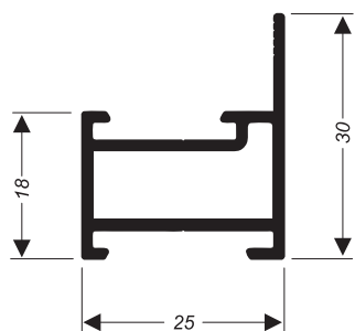
SU-080 (CX-149) 0,327 kg/m
