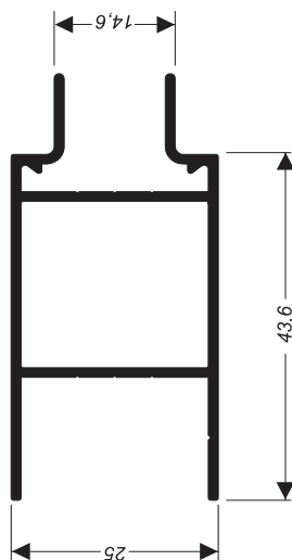
SU-191 0,533 kg/m
