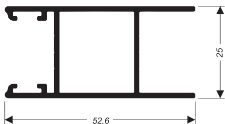
SU-068 (CX-341) 0,494 kg/m
