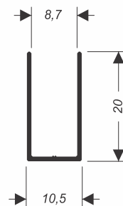
BX-110L 0,119 kg/m
