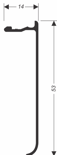
BX-265 0,197 kg/m
