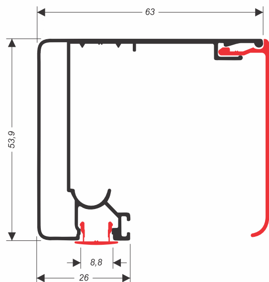
BX-283 0,715 kg/m
