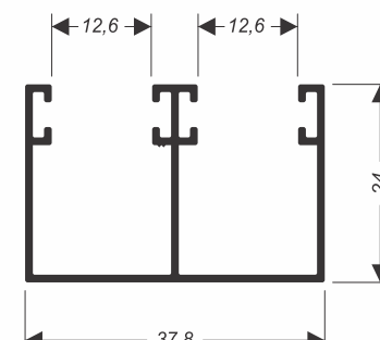
BX-282 0,360 kg/m
