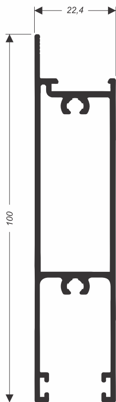
SU-225 (CX-343) 0,948 kg/m
