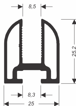
CEG-015 0,594 kg/m
