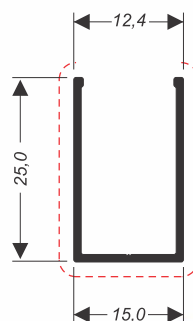
U-555L 0,171 kg/m
