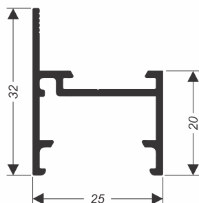
SU-088 0,316 kg/m
