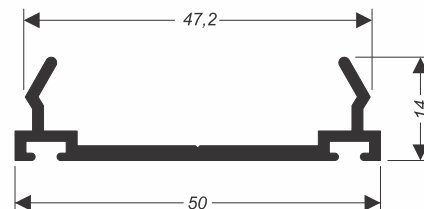
U-878 0,385 kg/m
