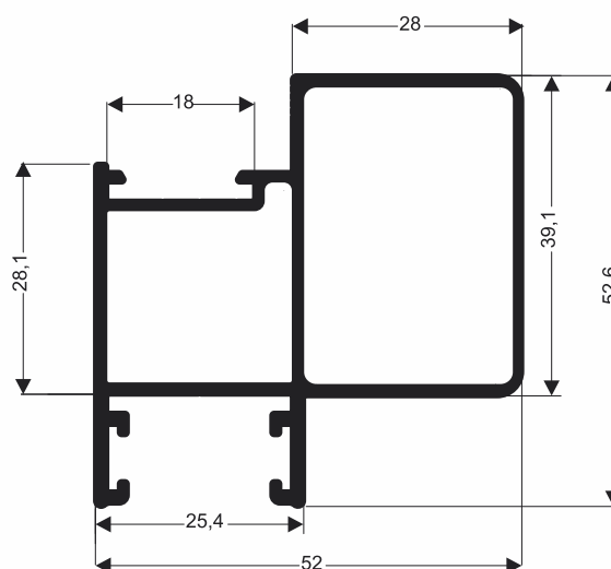
SU-044 0,981 kg/m
