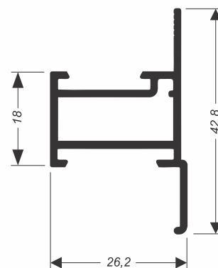
SU-081 (CX-150) 0,364 kg/m
