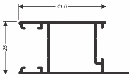
SU-039 (CX-154) 0,483 kg/m
