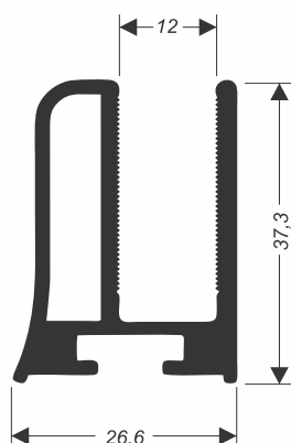
CEG-237 0,697 kg/m
