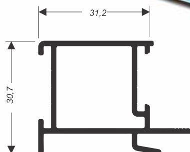
SU-040 (CX-155) 0,430 kg/m
