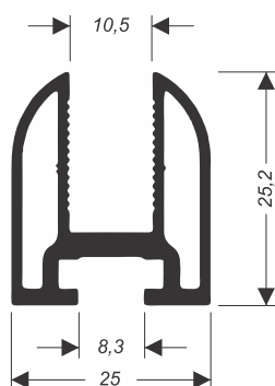
CEG-016 0,595 kg/m
