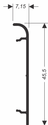
CEG-006 0,177 kg/m
