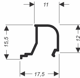
SU-102A 0,099 kg/m
