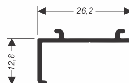
SU-084 0,116 kg/m
