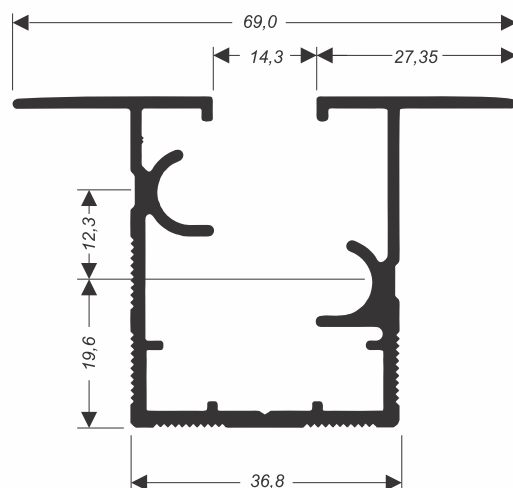
CEG-025 1,024 kg/m
