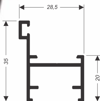
SU-079 (CX-342) 0,297 kg/m
