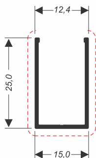
U-555L 0,171 kg/m
