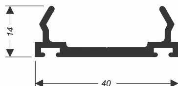
IFC-014 (U-615) 0,380 kg/m
