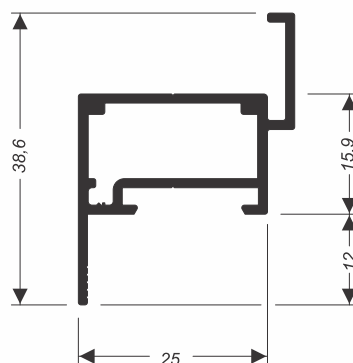
SU-098 0,401 kg/m
