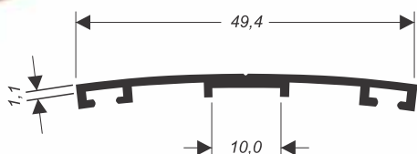
AL-1313 0,280 kg/m
