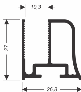
CEG-004 0,430 kg/m
