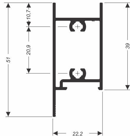
SU-110 0,534 kg/m
