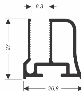
CEG-005 0,433 kg/m
