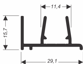
SU-008 (CX-333) 0,245 kg/m
