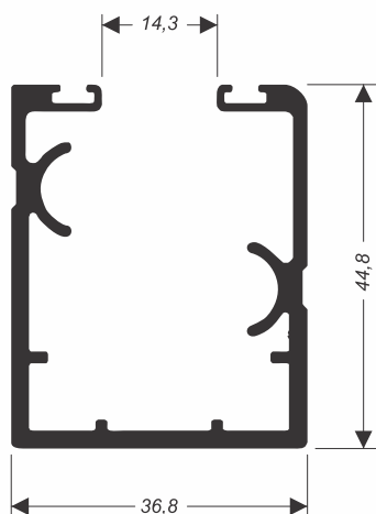
CEG-002 0,921 kg/m
