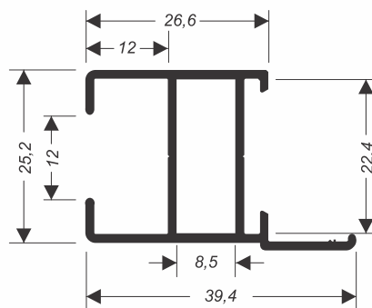
SU-090 0,380 kg/m
