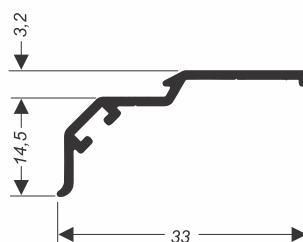
SU-083 (L-794) 0,145 kg/m
