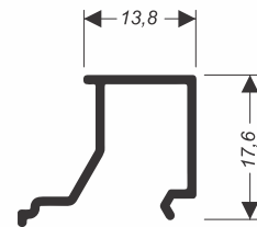
SU-103 (CX-145) 0,125 kg/m
