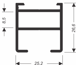
SU-091 0,401 kg/m
