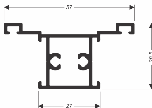
SU-086 (CX-146) 0,550 kg/m
