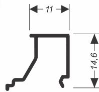
SU-102 (CX-144) 0,100 kg/m
