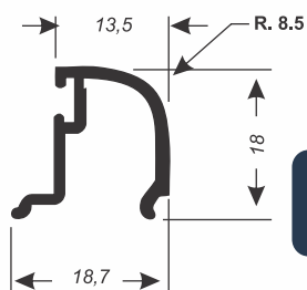
LG-026 0,158 kg/m
